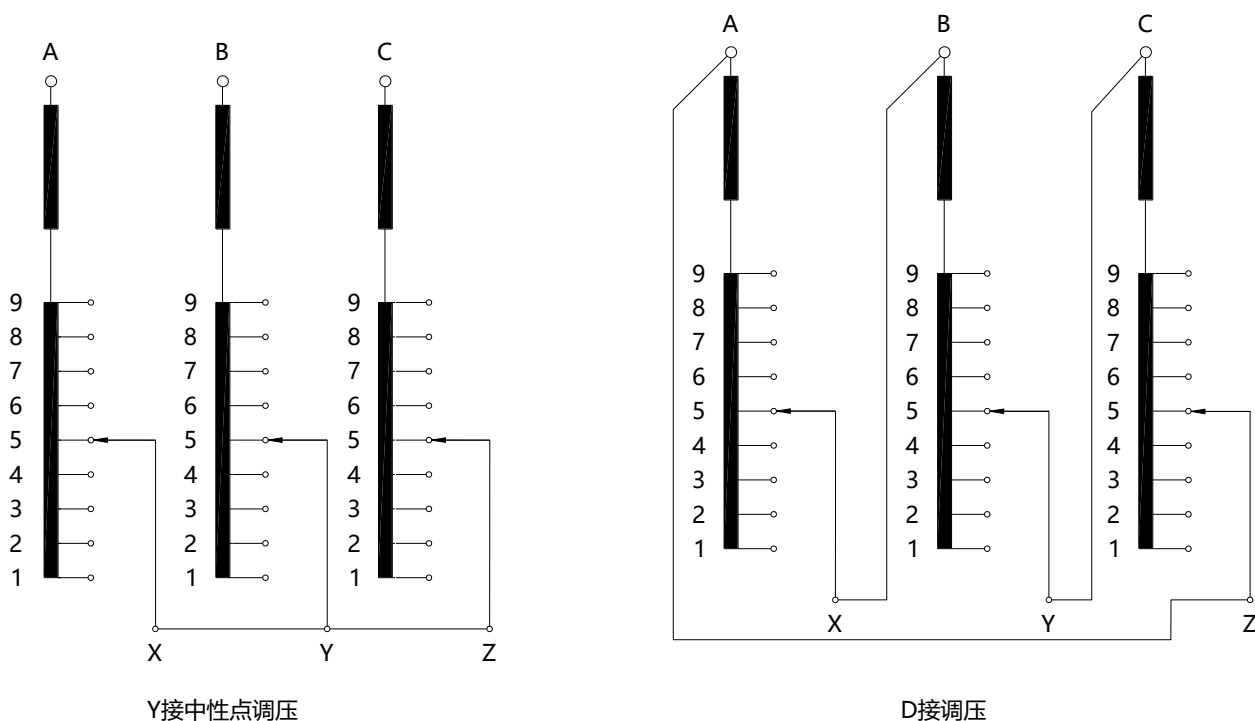
图 1-1 调压绕组的基本连接方式
