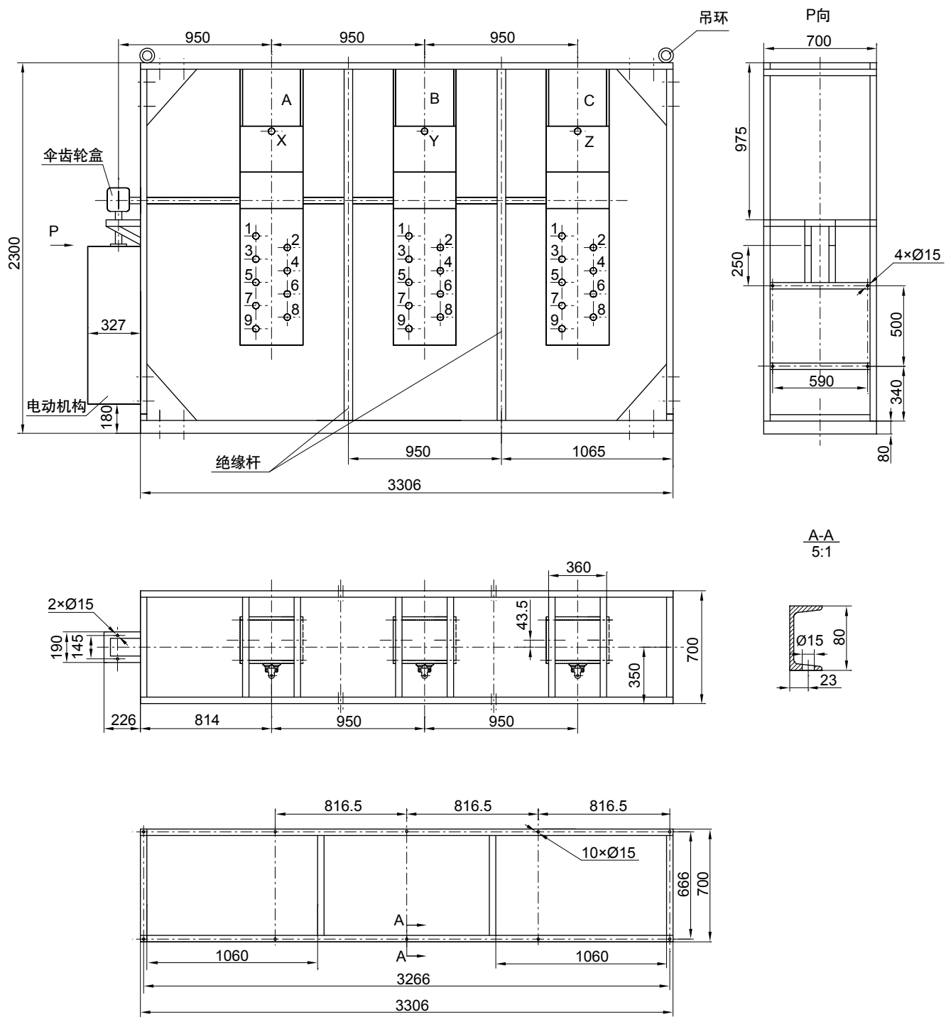
地基安装定位孔图
