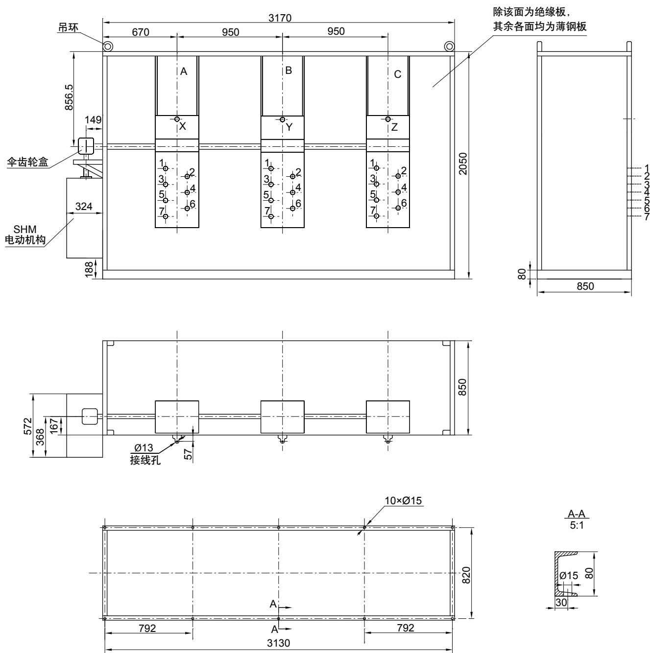
地基安装定位孔图
