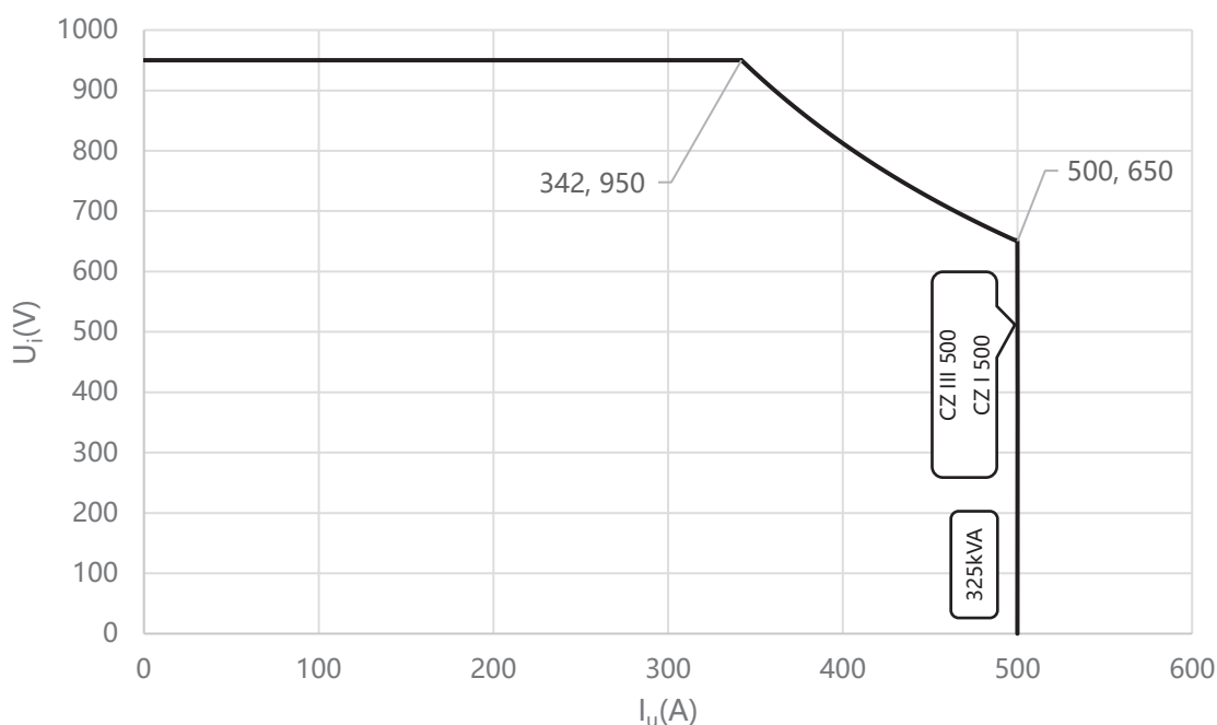
图 4-1 分接开关额定级容量
