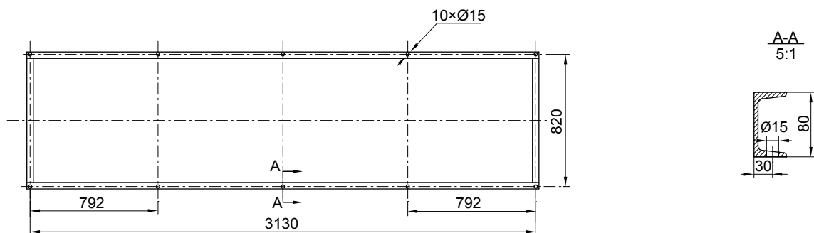
地基安装定位孔图
