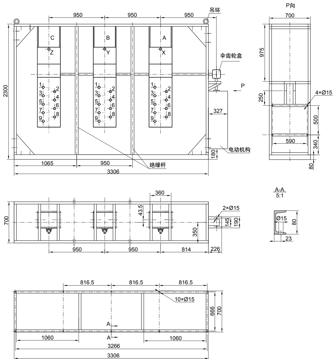
地基安装定位孔图
