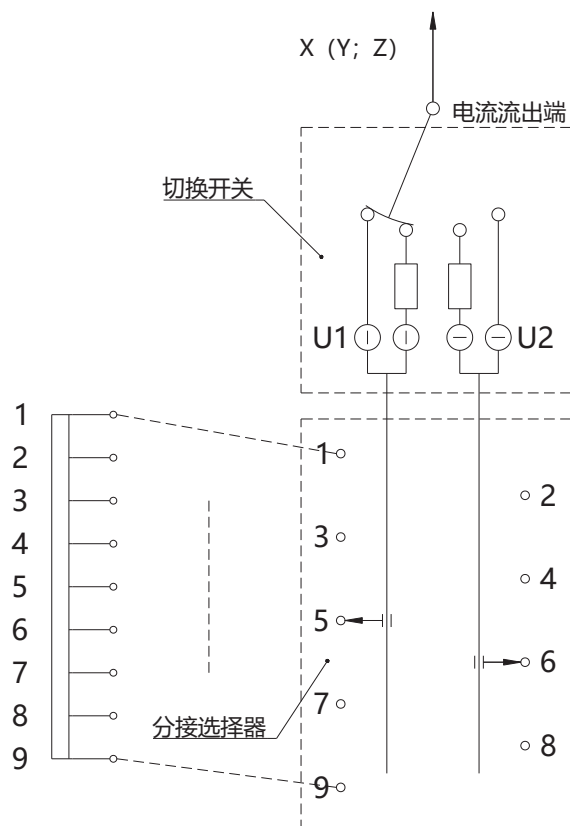
图 3-2 分接选择器基本接线图
