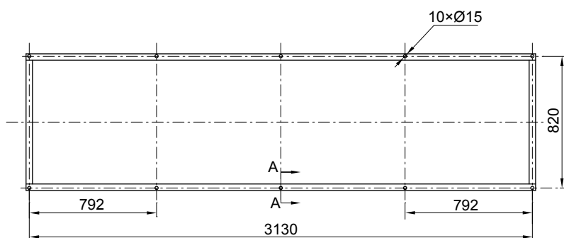
地基安装定位孔图
