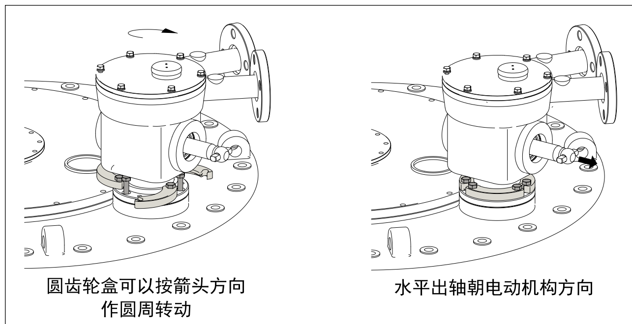
图 8-3 圆齿轮盒的调整与固定
