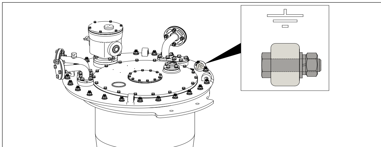
图 9-3 接地线连接
