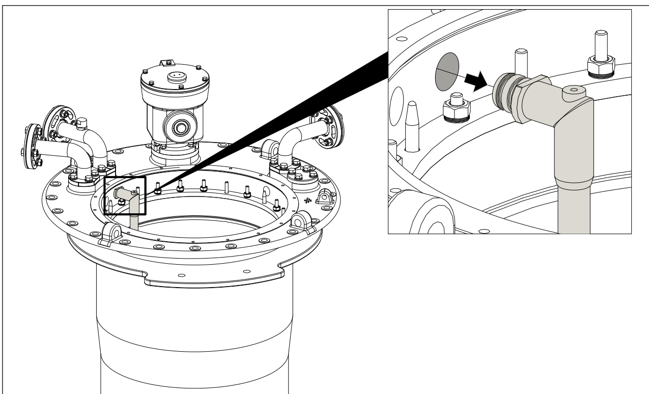
图 5-7 从 OLTC 安装法兰上拆除吸油管
