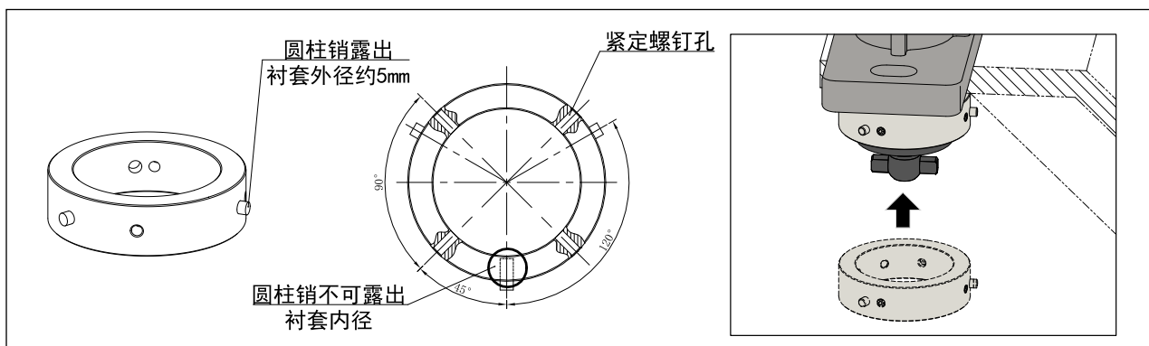
图 8-11 衬套安装
